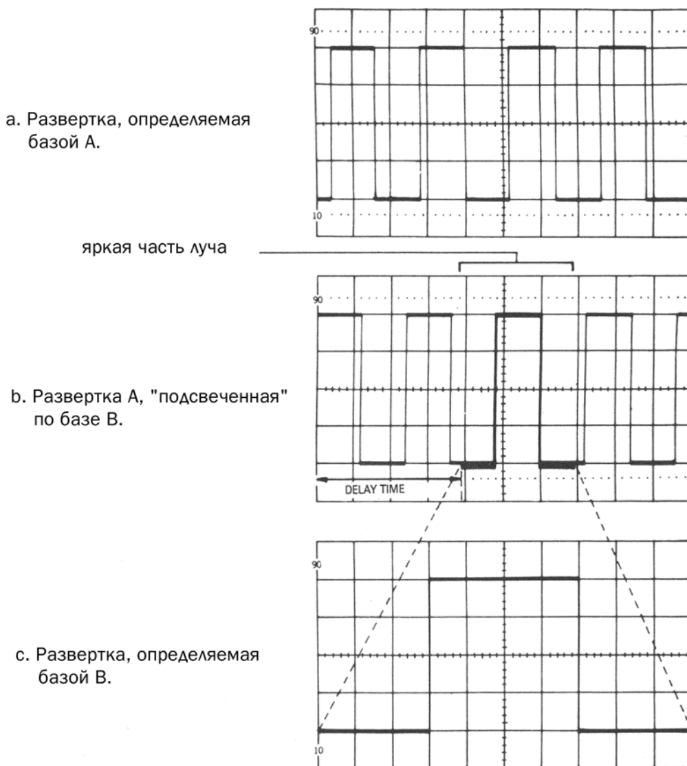
рис. 2-6. РАСТЯЖКА ИЗОБРАЖЕНИЯ С ИСПОЛЬЗОВАНИЕМ РАЗВЕРТКИ С ЗАДЕРЖКОЙ.
