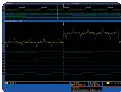
► Элементы управления Wave Inspector® значительно повышают эффективность перемещения по осциллограммам, их просмотра и анализа данных.
