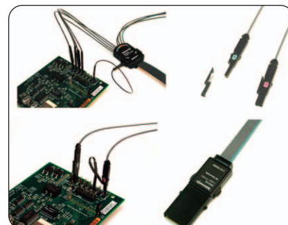
► Пробник P6516 для осциллографа смешанных сигналов.
