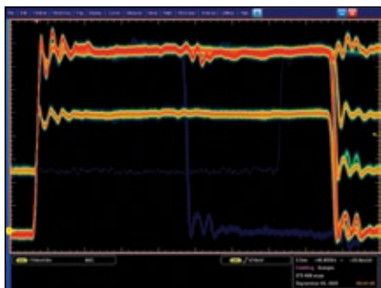
Режим захвата FastAcq максимально повышает вероятность регистрации глитчей и других редко происходящих событий
