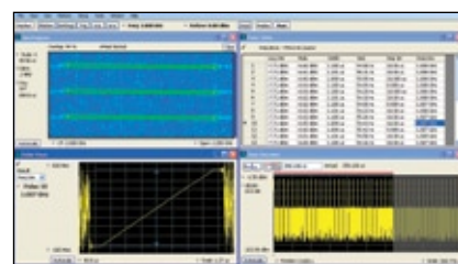
SignalVu™ предоставляет возможность подробного многодоменного анализа
