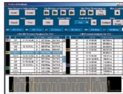
Измерение временных характеристики и декодирование протоколов CAN и LIN
