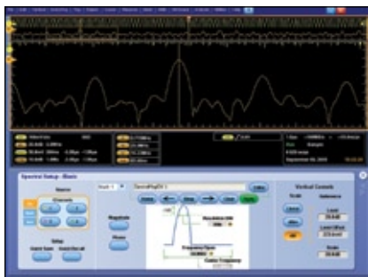
Базовое окно для отображения спектра
