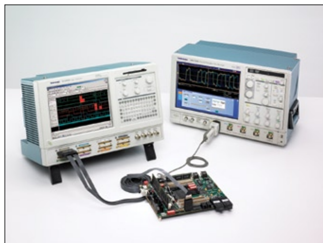
Интегрированный набор инструментов для проектирования и отладки цифровых схем
