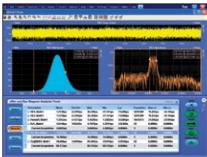
Анализ джиттера, временные характеристики и глазковая диаграмма
