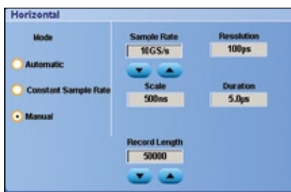
Три режима горизонтальной развертки
