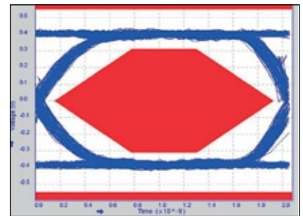
Проверка на совместимость для множества стандартов последовательных шин, таких как USB и Ethernet
