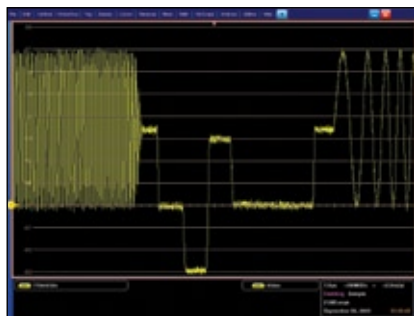
Запуск по аналоговому трехуровневому синхросигналу HDTV и анализ гасящего интервала строчной развертки
