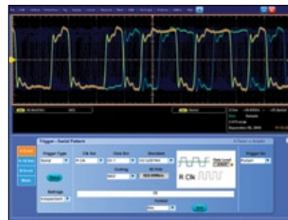
Запуск по заданной комбинации данных последовательной шины для отладки проблем, связанных с порядком следования данных
