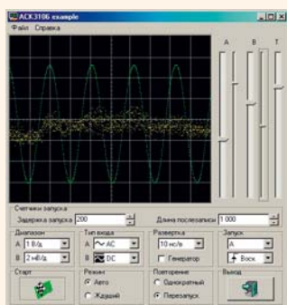
Окно примера приложения для Borland Builder
