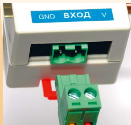
Рис. 2. Для подключения внешних соединений применяются легкоъемные винтовые терминалы
