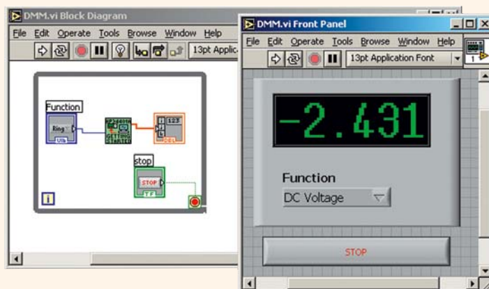
LabVIEW 3 программа цифрового мультиметра
