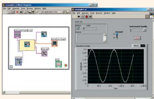
Использование APP-3007 в среде LabVIEW
