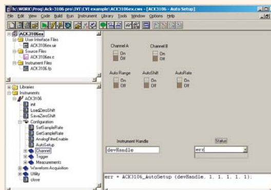
Использование функционального дерева инструмента в LabWindows/CVI
