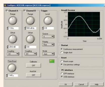
Диалоговая панель настройки экспресс-инструмента АСК-3106
